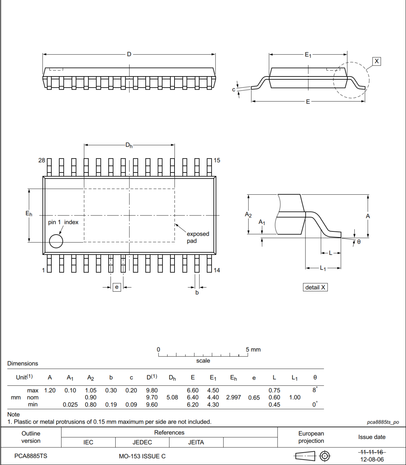
Fig 26. Package outline PCA8885TS (TSSOP28)
